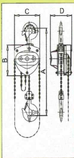
1-2-3- TON
