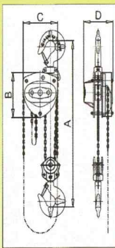
5 TON
