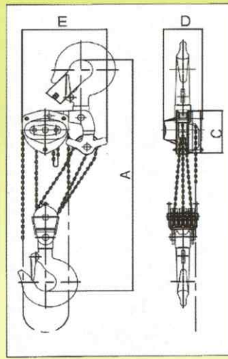
15 TON
