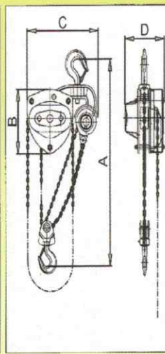
7.5 TON / 10 TON
